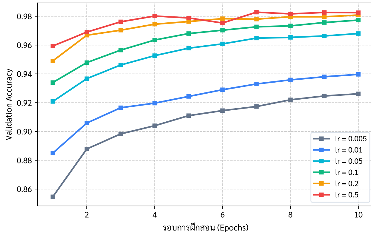
Validation Accuracy ตามอัตราการเรียนรู้ต่างๆ
