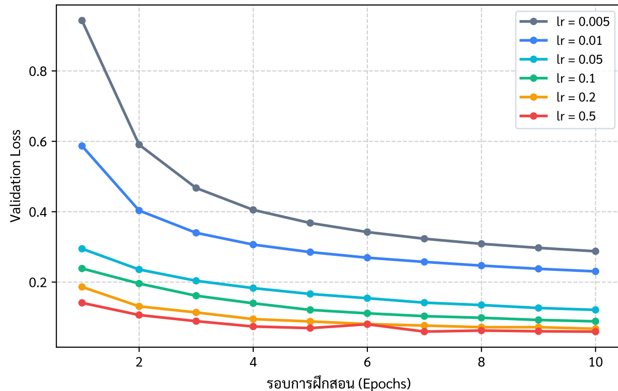
Validation Loss ตามอัตราการเรียนรู้ต่างๆ
